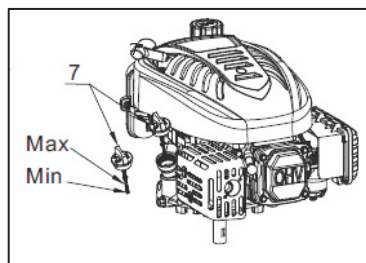
Abb. 7 7 Öleinfülldeckel/Ölmesstab Max: Obergrenze Min: Untergrenze
