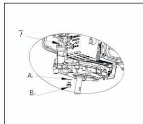
Abb. 8 7. Öleinfülldeckel/Ölmesstab A. Dichtungsring B. Ablassschraube
