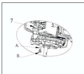
Fig. 8 7. Bouchon de remplissage d'huile / jauge A. Rondelle d'étanchéité B. Bouchon de vidange
