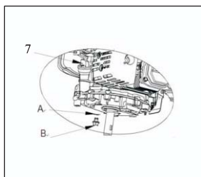
Fig. 8 7: Tappo/Asta graduata A: Guarnizione B: Vite di scarico
