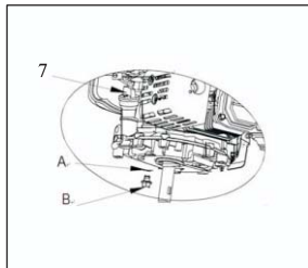
Fig. 8 7. Tapa del filtro de aceite/varilla de nivel A. Arandela de sellado B. Tornillo de drenaje
