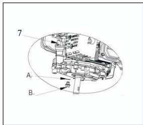
Abb. 8 7. Öleinfülldeckel/Ölmesstab A. Dichtungsschraube B. Ablassschraube
