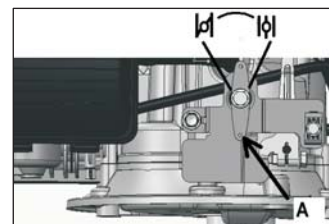
Abb. 2B A. Gashebel
