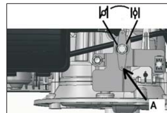
Fig. 2B A. Controlo do acelerador
