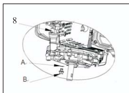
Fig. 8 8: Tappo/Asta graduata A: Guarnizione B: Vite di scarico
