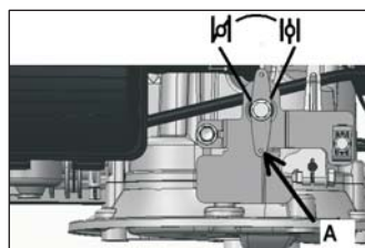
Fig. 2B A. Acceleratore
